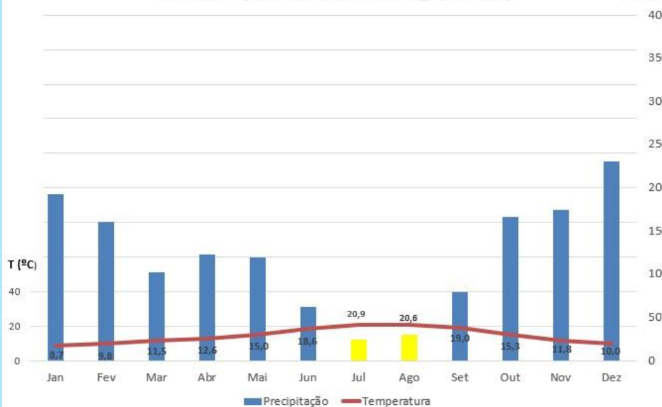
Gráfico termopluiométrico normal de Braga (1971-2000)
