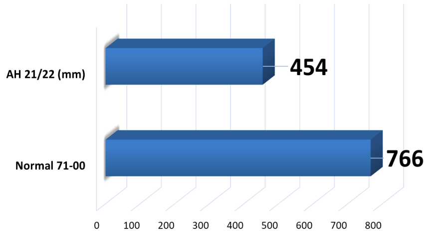
Precipitação acumulada (Out.21-Jan.22)
