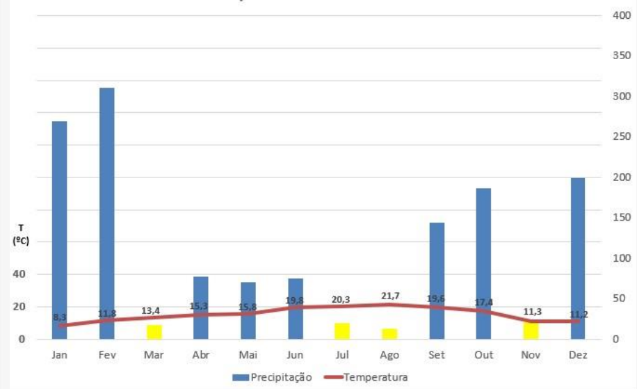
Gráfico termopluiométrico de Ponte de Lima - 2021
