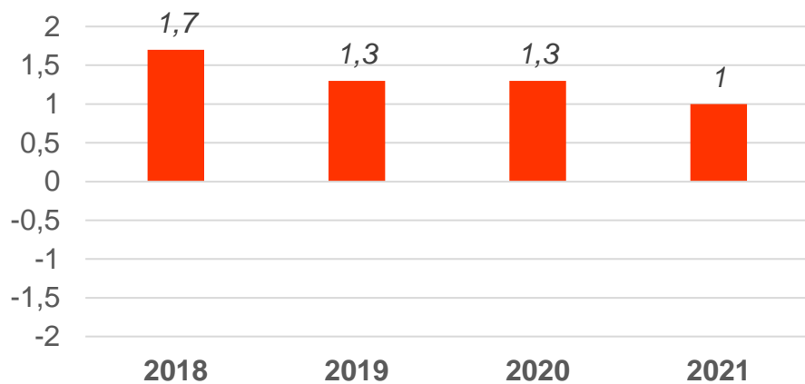
Variação (°c) da temperatura anual
