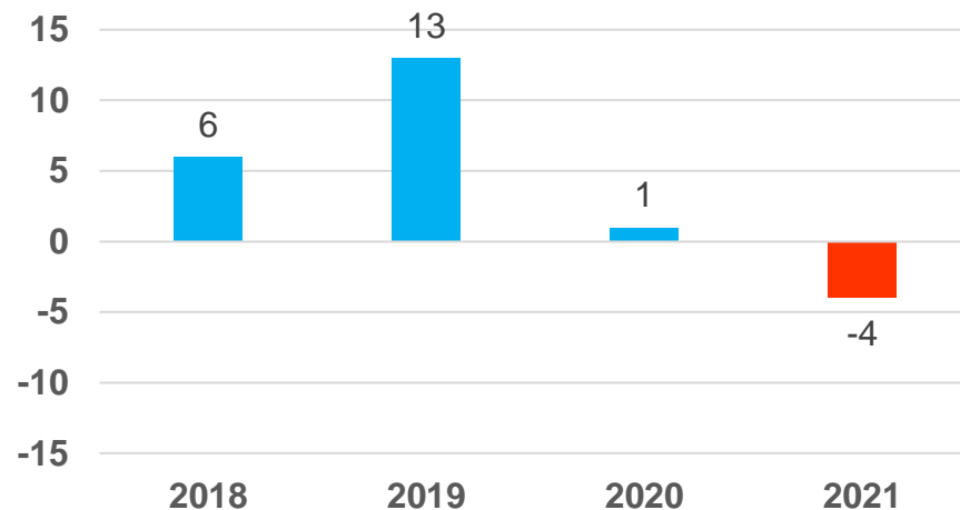
Variação (%) da precipitação anual
